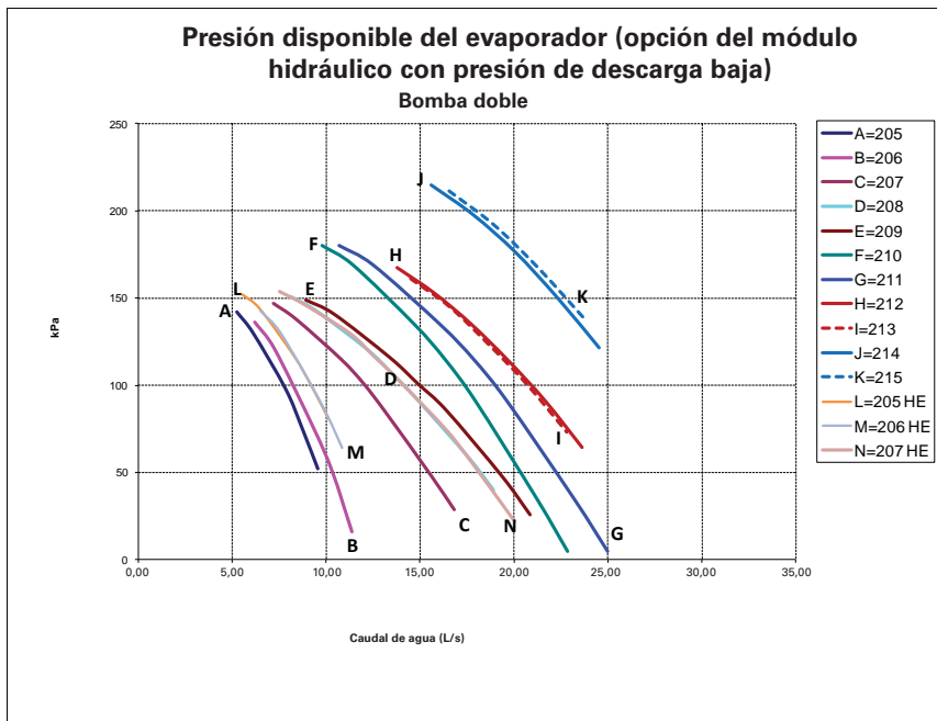
Ilustración 7: Presión disponible de la enfriadora; lado del evaporador; unidades de rendimiento estándar y alto rendimiento; presión de descarga baja; bomba doble
