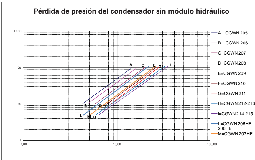
Ilustración 5: Pérdida de presión del condensador de las unidades estándar
