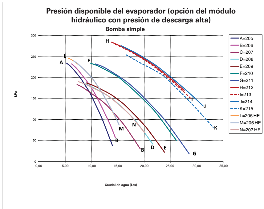
Ilustración 8: Presión disponible de la enfriadora; lado del evaporador; unidades de rendimiento estándar y alto rendimiento; presión de descarga alta; bomba simple
