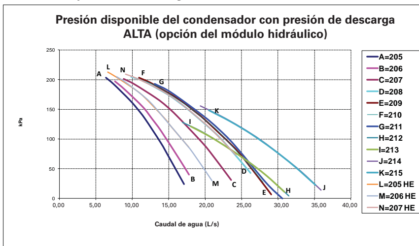
Ilustración 11: Presión disponible de la enfriadora; lado del condensador; unidades de rendimiento estándar y alto rendimiento; presión de descarga alta
