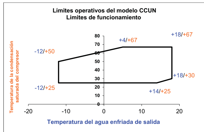
Ilustración 2: Límites de funcionamiento del modelo CCUN
