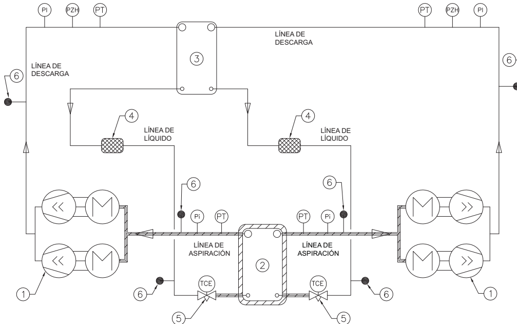
Ilustración 13: Gráfico del caudal de refrigerante del modelo CGWN (212-215)
