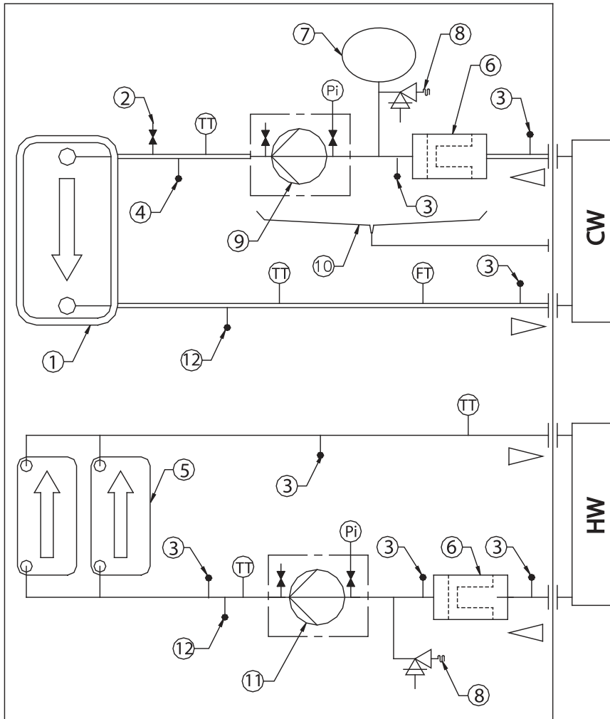
Ilustración 21: Gráfico del caudal hidráulico del modelo CGWN con módulo hidráulico (212-215)
