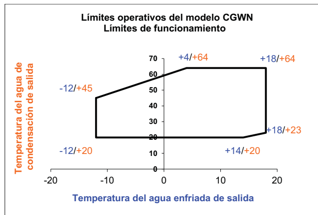
Ilustración 1: Límites de funcionamiento del modelo CGWN
