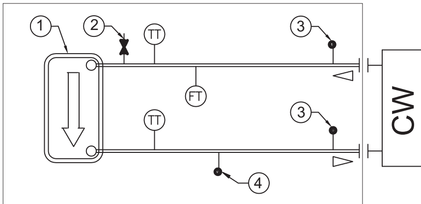
Ilustración 18: Gráfico del caudal hidráulico del modelo CCUN sin módulo hidráulico (205-211)
