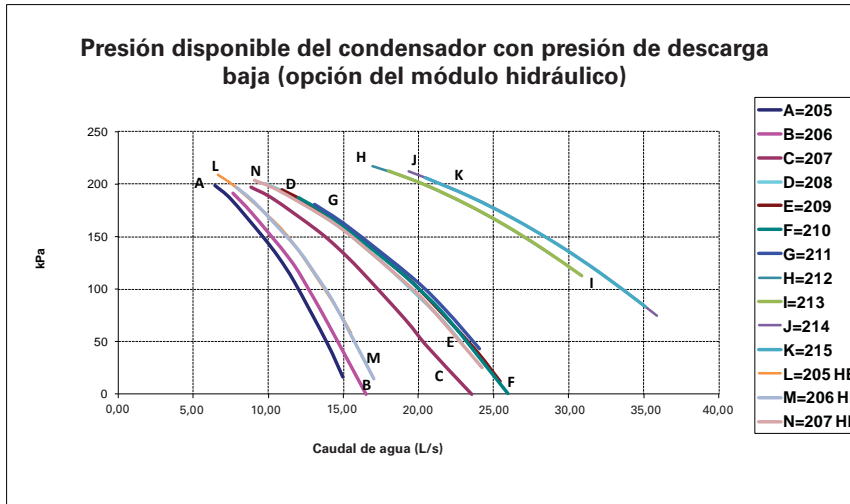
Ilustración 10: Presión disponible de la enfriadora; lado del condensador; unidades de rendimiento estándar y alto rendimiento; presión de descarga baja
