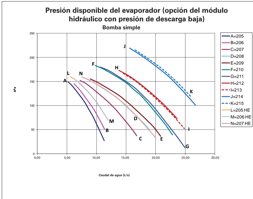
Ilustración 6: Presión disponible de la enfriadora; lado del evaporador; unidades de rendimiento estándar y alto rendimiento; presión de descarga baja; bomba simple
