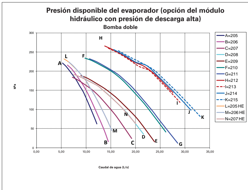
Ilustración 9: Presión disponible de la enfriadora; lado del evaporador; unidades de rendimiento estándar y alto rendimiento; presión de descarga alta; bomba doble
