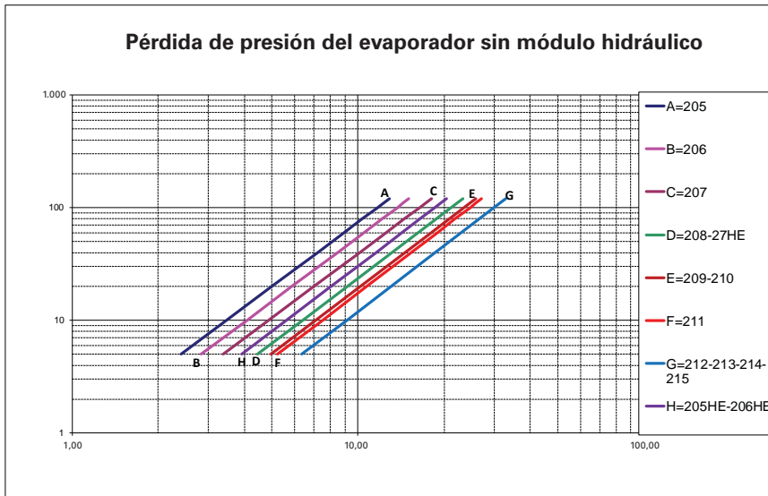
Ilustración 4: Pérdida de presión del evaporador de las unidades de rendimiento estándar y alto rendimiento
