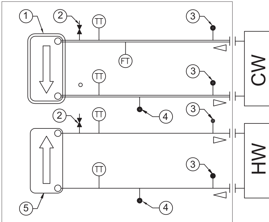
Ilustración 16: Gráfico del caudal hidráulico del modelo CGWN sin módulo hidráulico (205-211)
