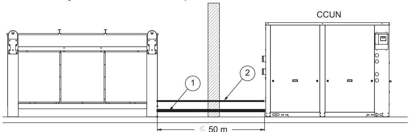
Ilustración 3: Configuración de la instalación: CCUN y unidad de condensación remota al mismo nivel
